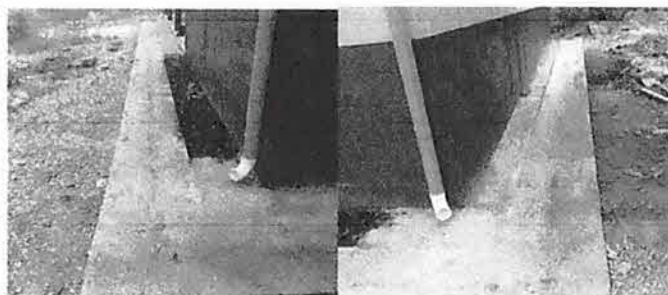
Foto 11: Reemplazamiento de Cuneta fundida de 60 cm X 0.10 cm de espesor.
